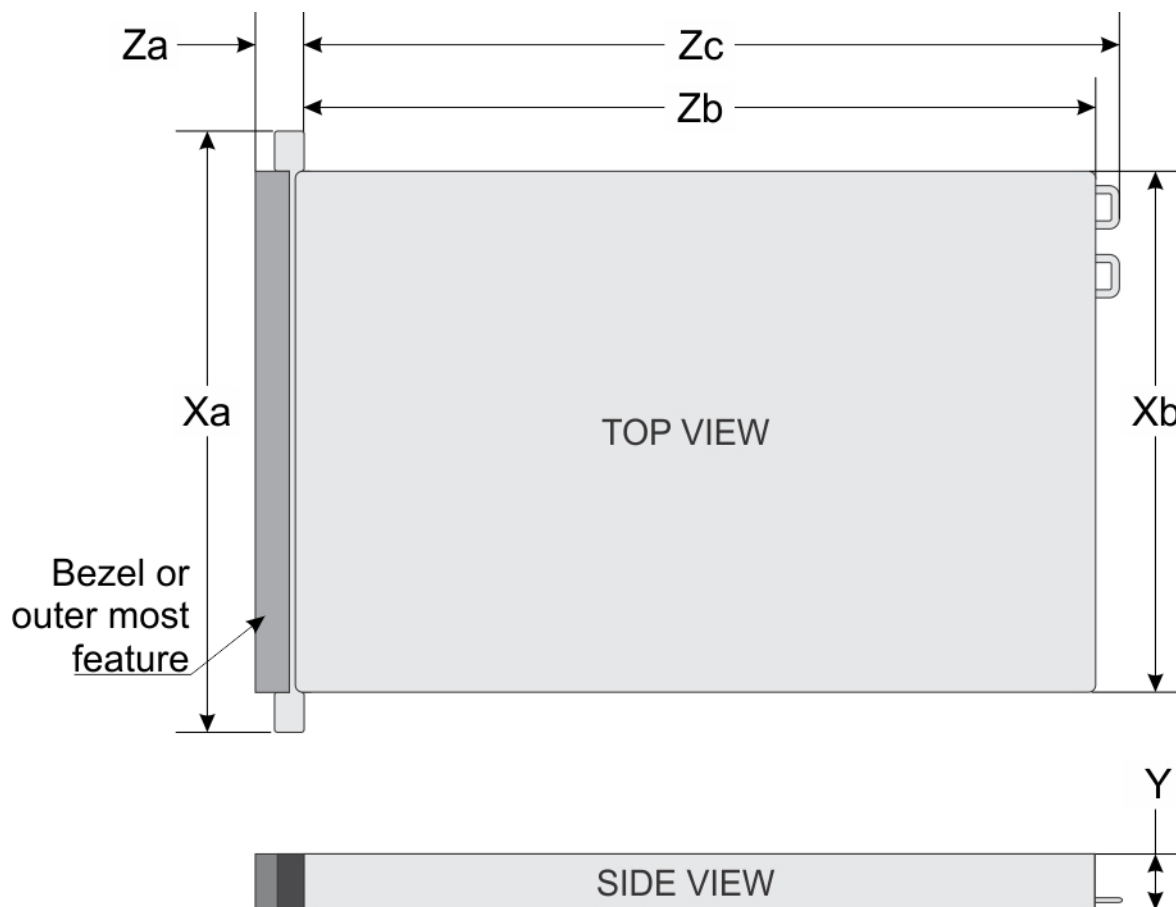
図 13. システムの寸法
