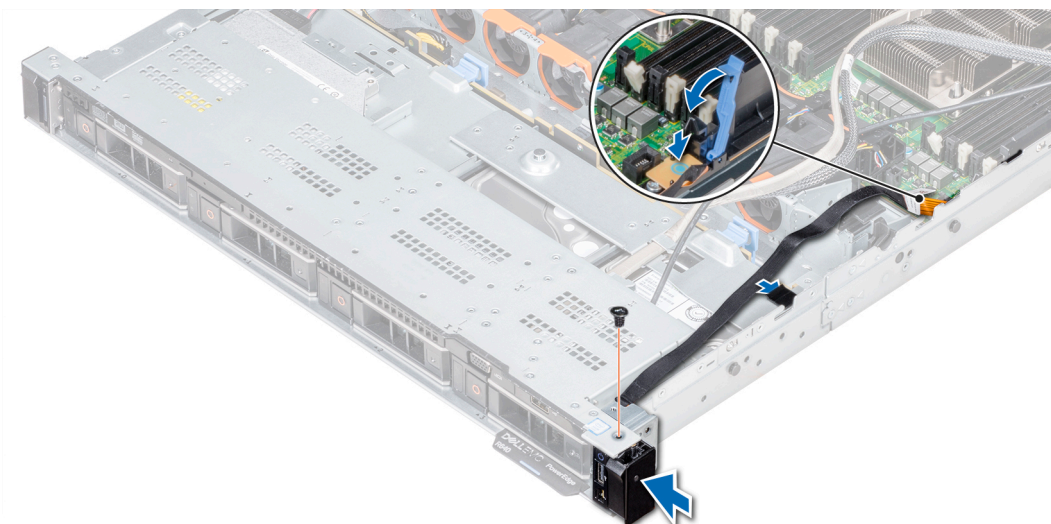
図 81. 右のコントロールパネルの取り付け
