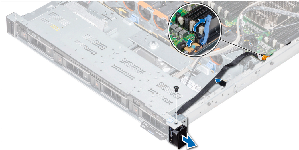
図 80. 右コントロールパネルの取り外し
