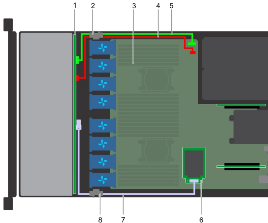
図 63. ケーブル配線 - 3.5 インチ ( x4 ) ハードドライブバックプレーン
