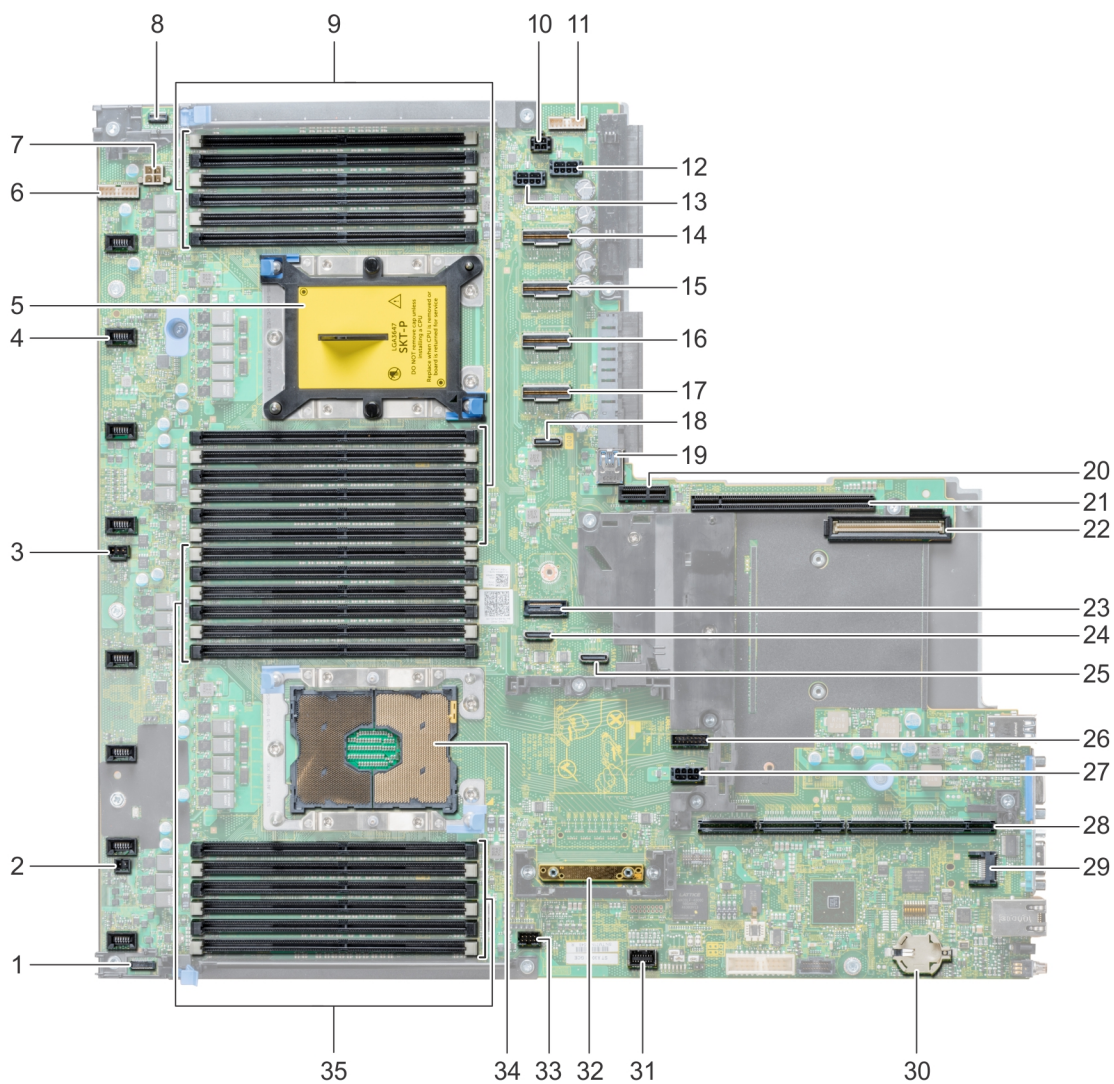
図 83. システム基板のジャンパとコネクタ
