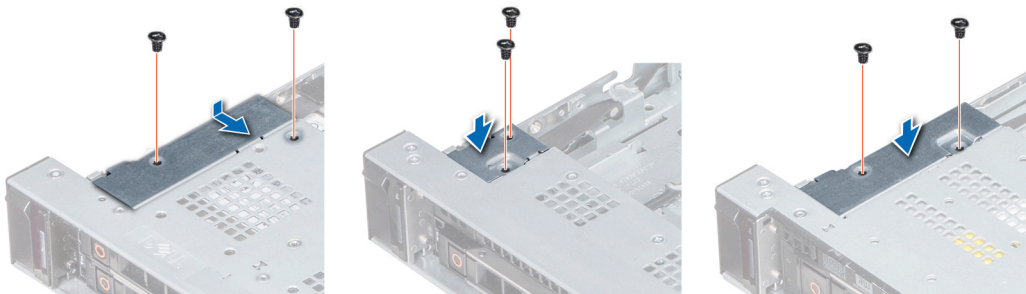
図 78. ケーブルカバーの取り付け
