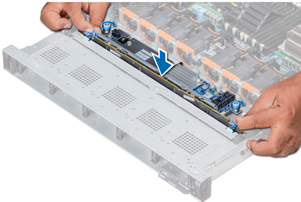
図 61. ハードドライブバックプレーンの取り付け
