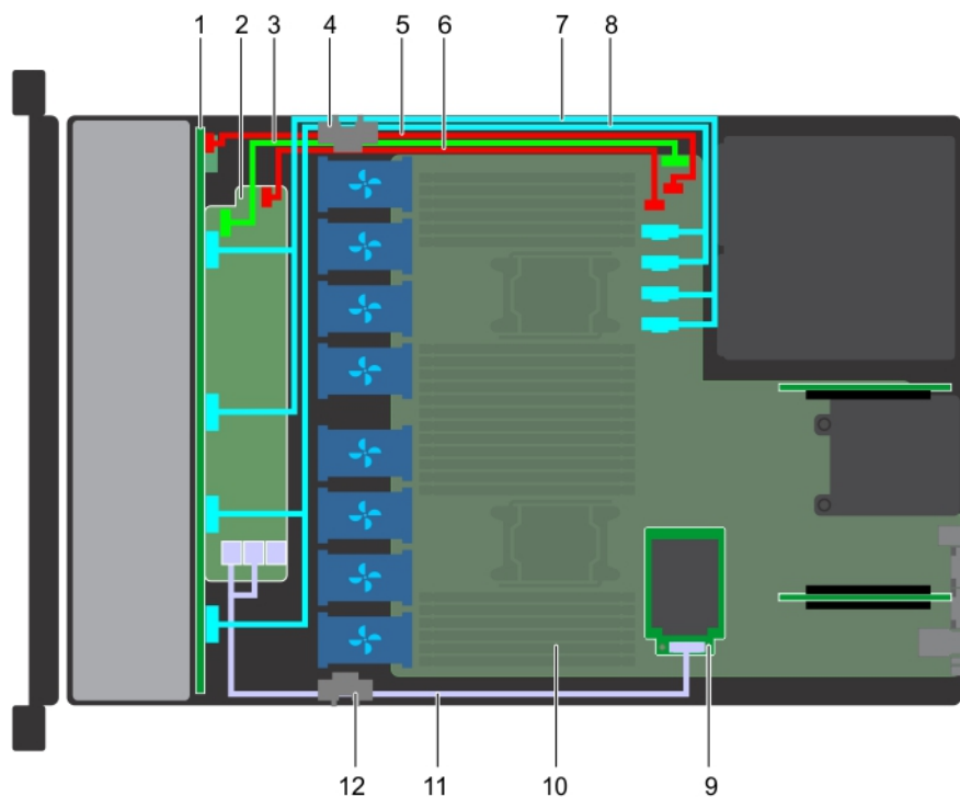
図 62. ケーブル配線 - 2.5 インチ (x10) ハードドライブバックプレーン
