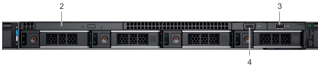
図 2. 4 x 3.5 インチドライブシステムの正面図
