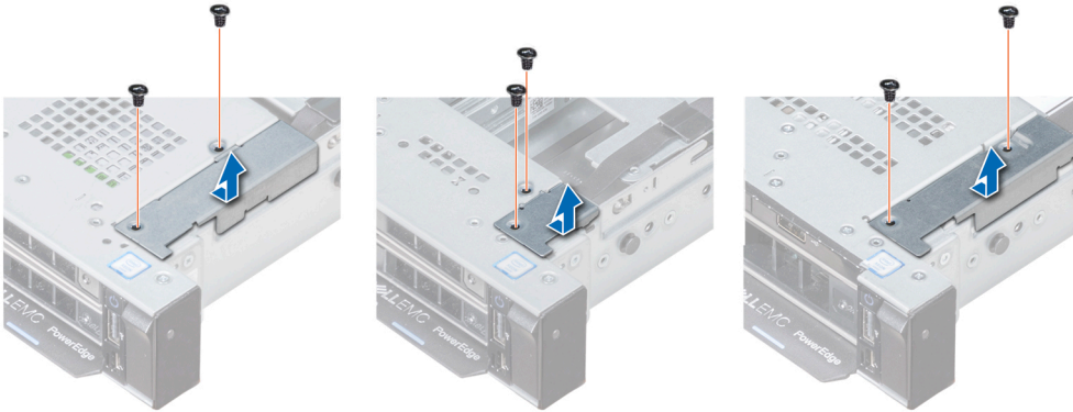
図 79. ケーブルカバーの取り外し
